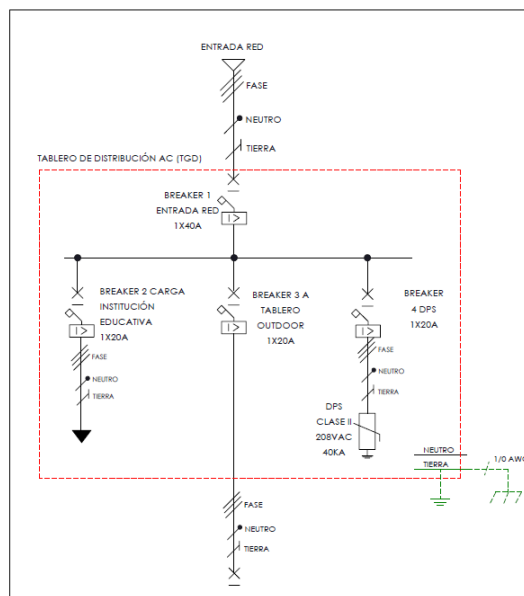
Posible Diagrama unifilar
